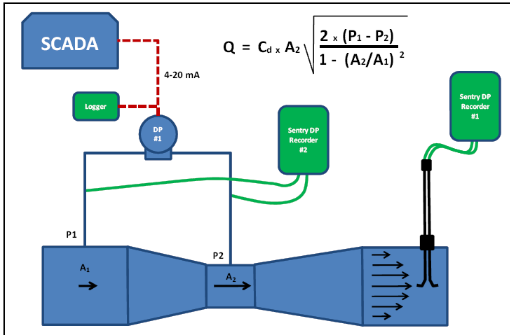
Fig. 1 – Venturi Meter Test Set Up
